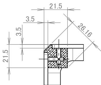
断面図 A-A
