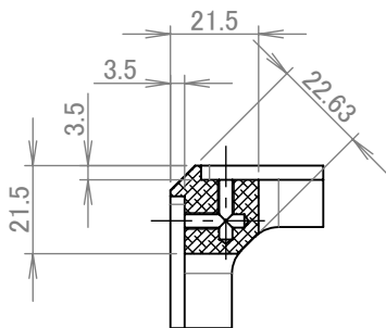
断面図 B-B
