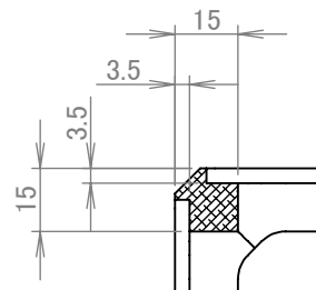
断面図 A-A
