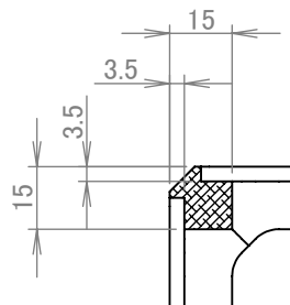
断面図 B-B
