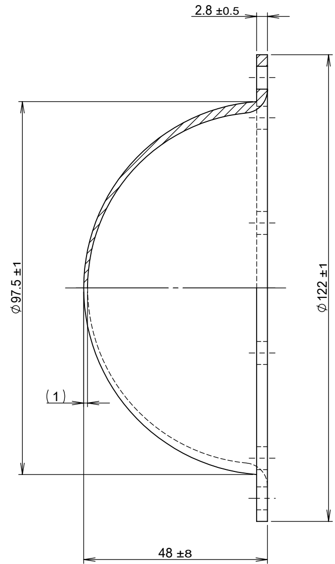
断面図 A-A
