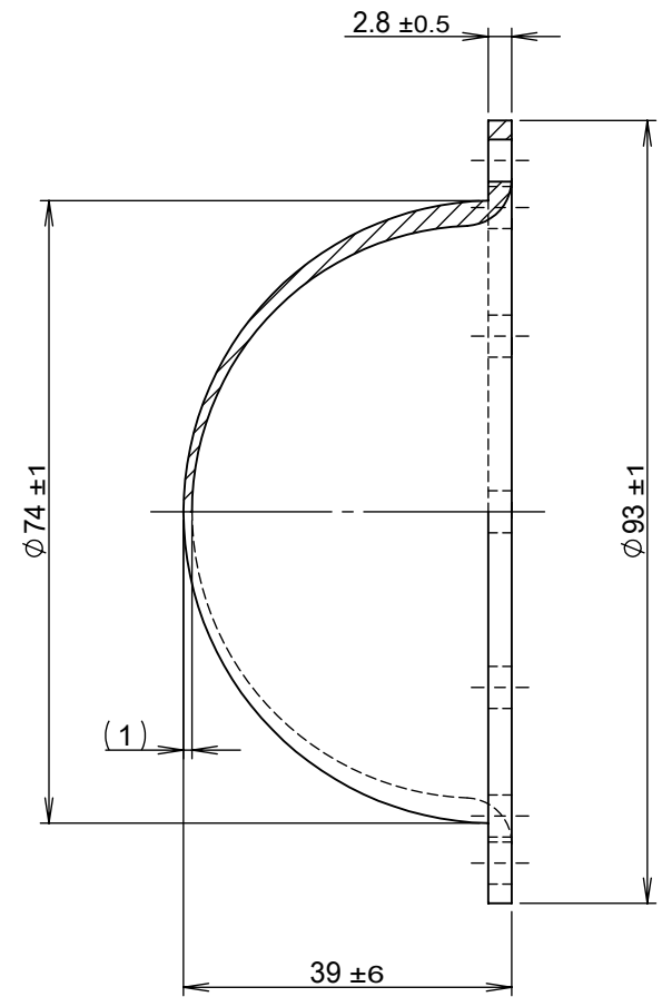
断面図 A-A
