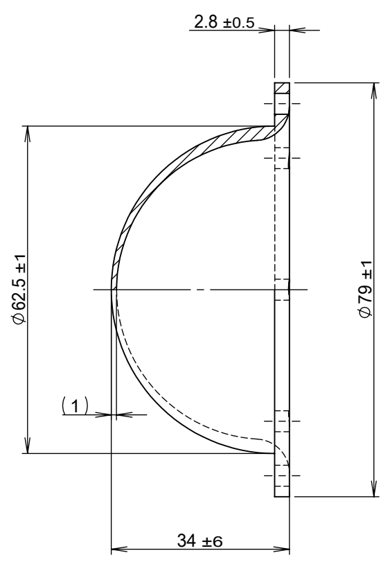
断面図 A-A
