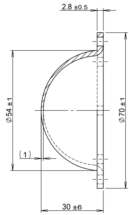
断面図 A-A
