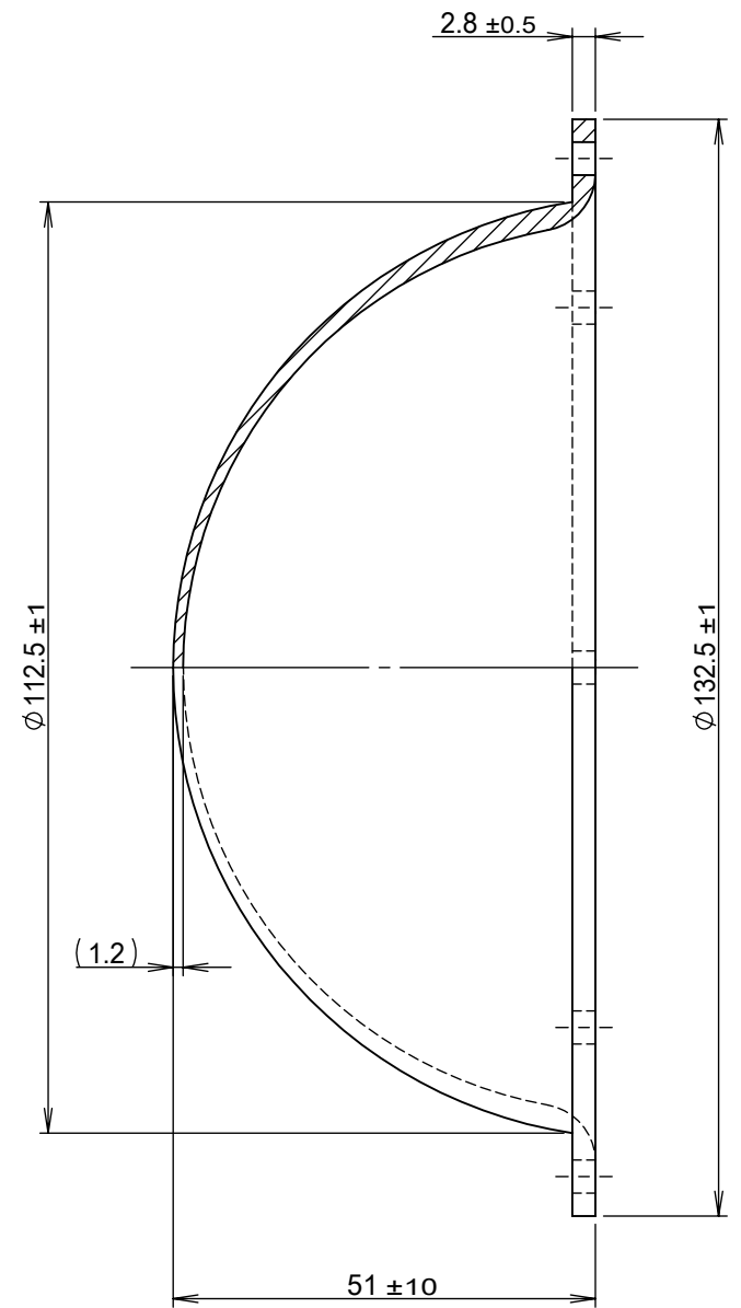
断面図 A-A
